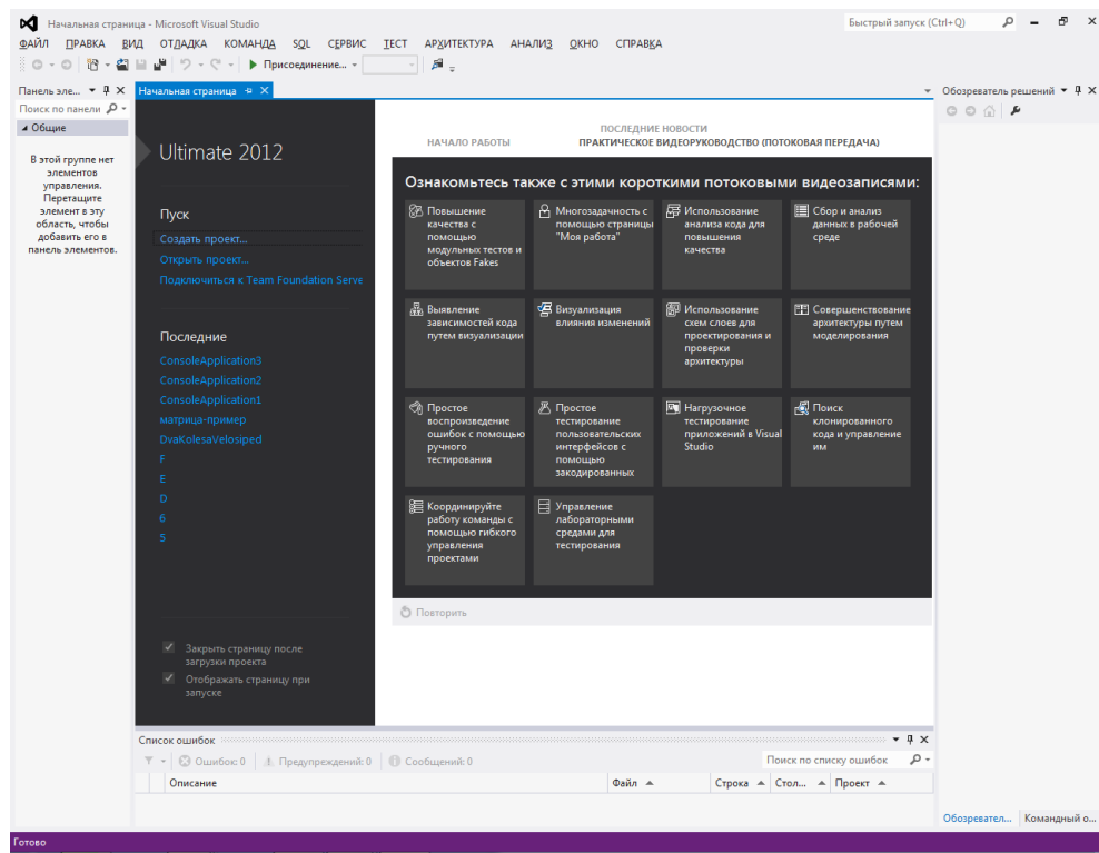
Рис. 5. Начальная страница.
