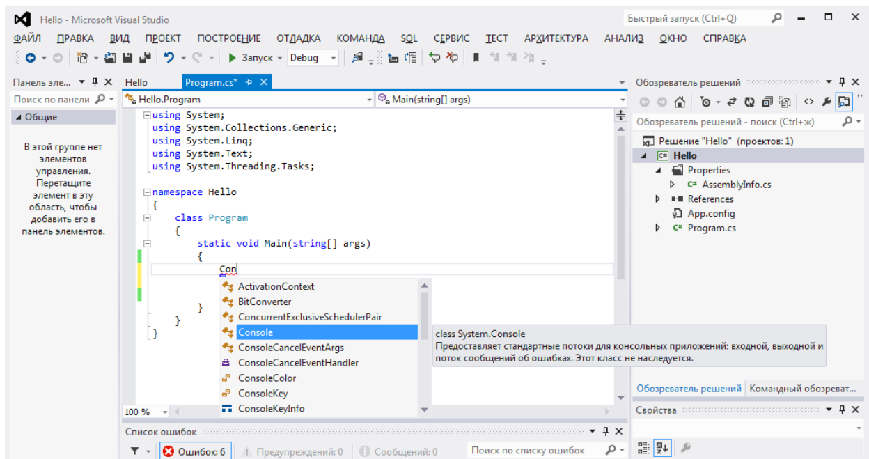
Рис. 9 . Технология IntelliSense
