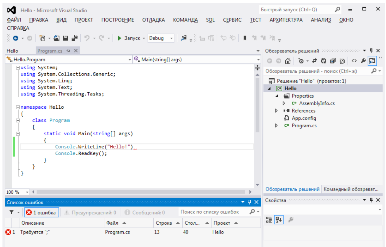
Рис. 12. Отладка ошибок.
