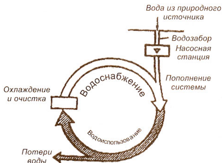
Рисунок 3.2 – Схема оборотного водоснабжения
