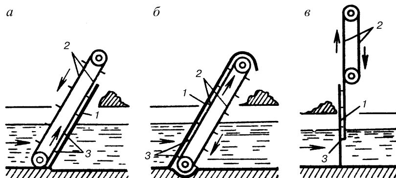
Рисунок 5.3 - Виды решеток с граблями для очистки: 1 – решетка; 2 – бесконечная цепь; 3 – грабли
