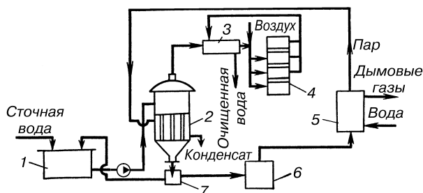
Рис. 5.17 - Схема установки для очистки сточных вод каталитическим окислением: 1 – емкость; 2 – выпарной аппарат; 3 – теплообменник; 4 – контактный аппарат; 5 – котел-утилизатор; 6 – печь; 7 – центрифуга
