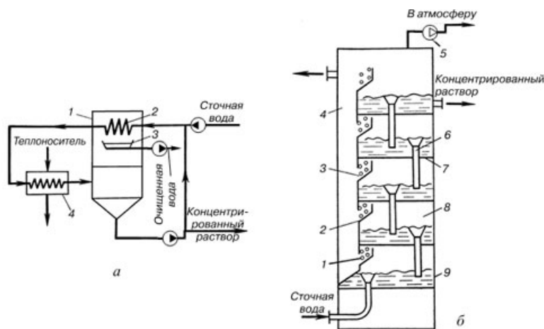
Рисунок 5.13 - Схемы адиабатных испарительных установок: а – одноступенчатой: 1 – камера испарения; 2 – конденсатор; 3 – поддон; 4 – подогреватель; б – вертикальной: 1 – конденсатор; 2 – желоб; 3 – канал для отвода конденсата; 4 – вертикальный канал; 5 – вакуумный насос; 6 – переточная труба; 7 – перегородка; 8 – испарительная камера; 9 – корпус
