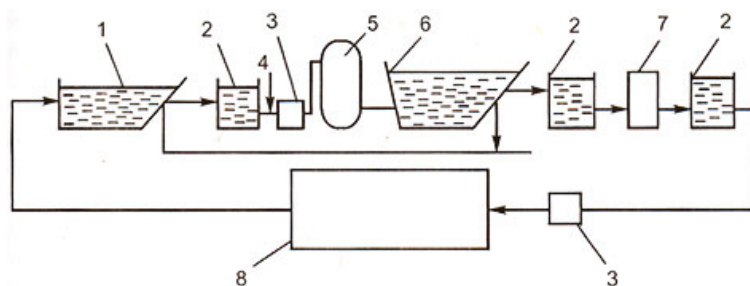
Рисунок 3.4 – Схема оборотного водоснабжения прокатного стана
