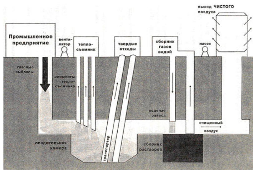
Рисунок 4.6 – Подземная универсальная система утилизации
