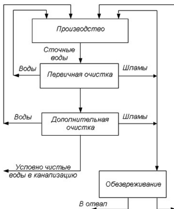
Рисунок 5.2 – Типовая схема очистки сточных вод
