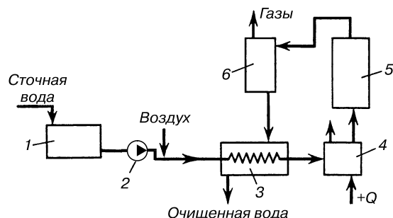
Рис. 5.16 - Схема установки для жидкофазного окисления: 1 – сборник; 2 – насос; 3 – теплообменник; 4 – печь; 5 – реактор; 6 – сепаратор
