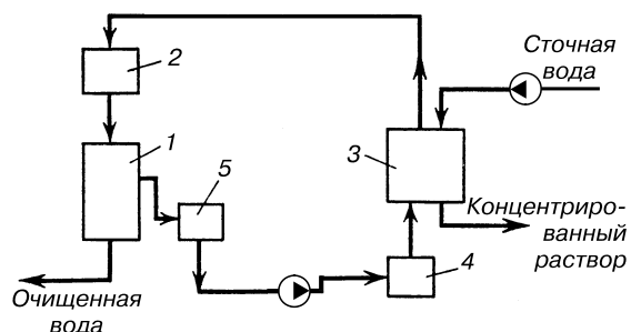
Рисунок 5.15 - Схема установки для очистки воды методом гидратообразования: 1 – сепаратор; 2 – камера плавления; 3 – камера гидратообразования; 4 – емкость; 5 – конденсатор
