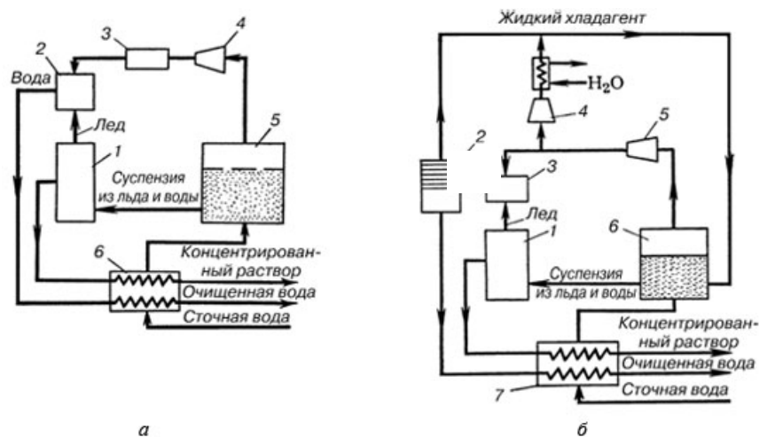
Рисунок 5.14 - Схемы установок концентрирования растворов вымораживанием: а – под вакуумом: 1 – промывная колонна; 2 – конденсатор-плавитель; 3 – вспомогательная холодильная установка; 4 – компрессор; 5 – кристаллизатор; 6 – теплообменник; б – при контактом вымораживании: 1 – промывная колонна; 2 – смеситель; 3 – конденсатор-плавитель; 4 – вспомогательный компрессор; 5 – главный компрессор; 6 – кристаллизатор; 7 – теплообменник
