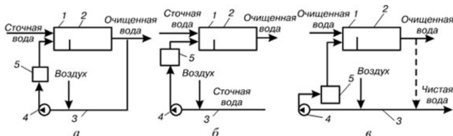
Рисунок 5.8 - Схемы подачи воды при напорной флотации: а – с рециркуляцией; б – с частичной подачей воды насосом; в – с рабочей жидкостью; 1 – приемные отделения; 2 – флотационные отделения; 3 – линии всасывания; 4 – насосы; 5 – напорные баки
