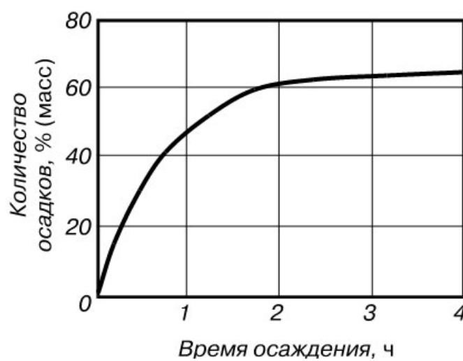
Рисунок 5.5 - График кинетики процесса осаждения
