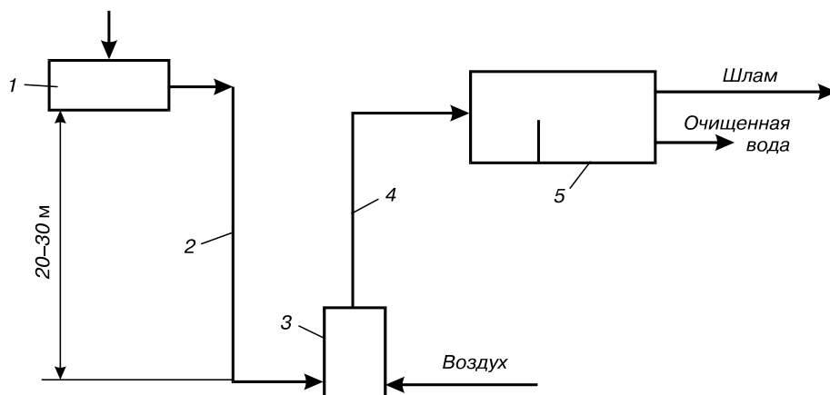
Рисунок 5.9 - Схема эрлифтной установки: 1 – емкость; 2 – трубопровод; 3 – аэратор; 4 – труба эрлифта; 5 – флотатор
