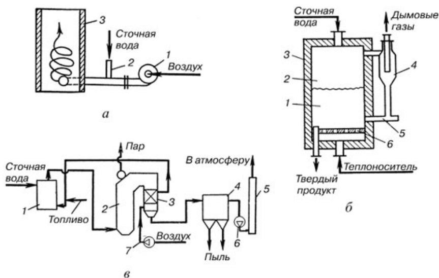
Рисунок 5.18 - Схемы устройств для огневого обезвреживания сточных вод: а – циклонная печь: 1 – воздухоподогреватель; 2 – питающее устройство; 3 – печь; б – печь с псевдоожиженным слоем: 1 – плотная фаза ожиженного слоя; 2 – разбавленная фаза; 3 – печь; 4 – циклон; 5 – труба для возврата материала; 6 – газораспределительная решетка; в – печь с котлом-утилизатором: 1 – печь; 2 – котел-утилизатор; 3 – воздухоподогреватель; 4 – аппарат сухой очистки газов; 5 – труба; 6 – дымосос; 7 – воздухоподогреватель
