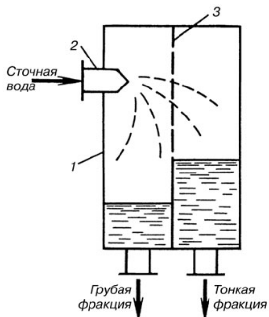
Рисунок 5.4 - Фракционер: 1 – корпус; 2 – сопло; 3 – сетка
