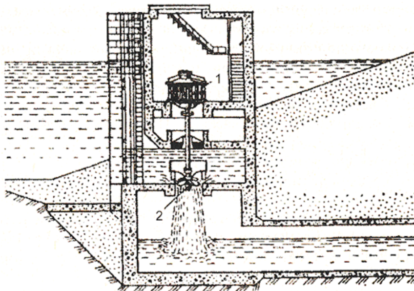
Рисунок 4.2 – Схема МГЭС с вертикальной пропеллерной турбиной: 1 – генератор; 2 – турбина
