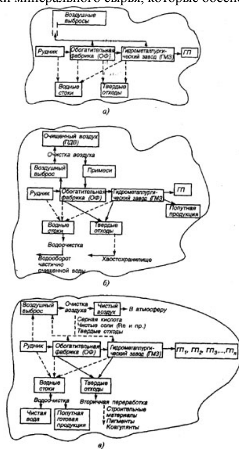
Рисунок 1.5 – Схемы добычи и переработки минерального сырья: а – открытой; б – полуоткрытой; в – закрытой системах; ГП – готовая продукция
