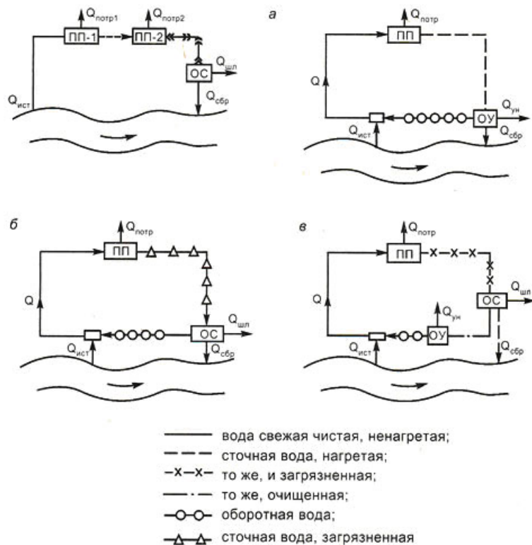
Рисунок 3.3 – Схема оборотного водообеспечения промышленных предприятий: а) с охлаждением; б) с очисткой; в) с очисткой и охлаждением (А.Ф. Порядин, А.Д. Хованский, 1996 г.)
