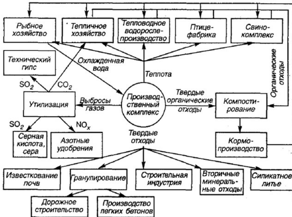
Рисунок 3.1 – Принципиальная схема безотходного промышленного производства
