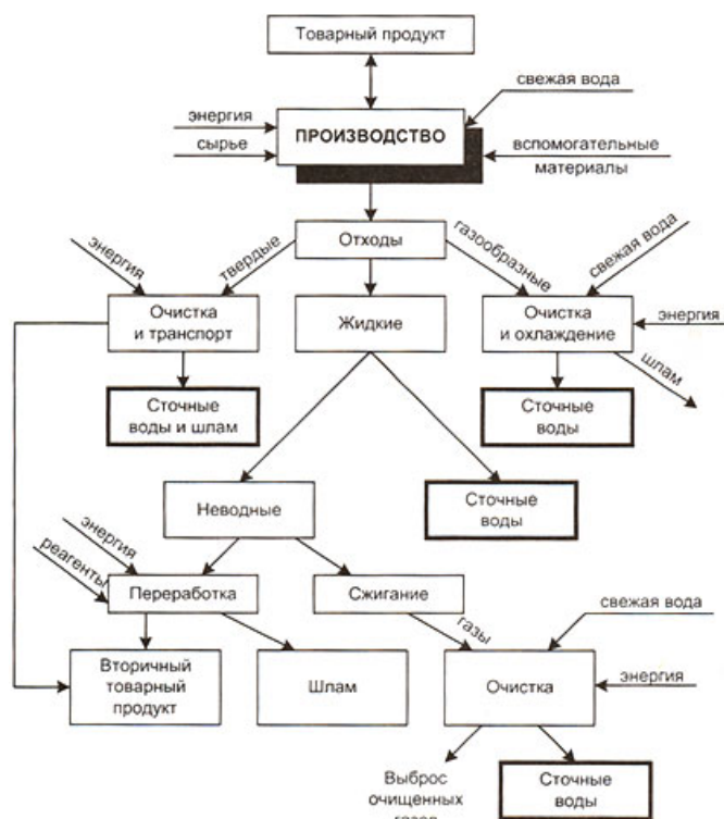
Рисунок 5.1 – Схема образования сточных вод в процессе материального производства
