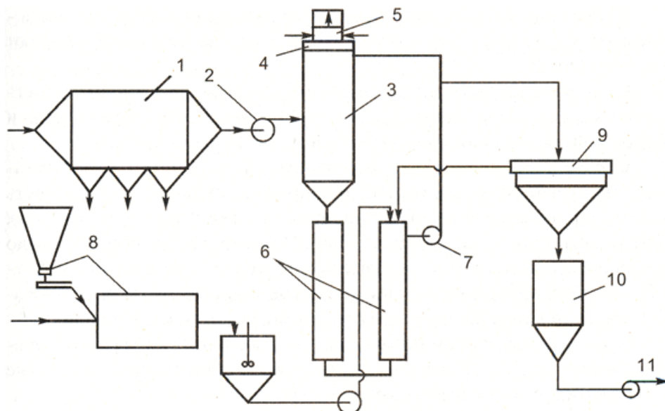
Рисунок 4.5 – Принципиальная схема очистки дымовых газов с \text{SO}_2 известняковым способом: 1 – золоуловитель; 2 – дымосос; 3 – скруббер; 4 – брызгоуловитель; 5 – подогреватель; 6 – емкости; 7 – циркуляционный насос; 8 – установка для приготовления суспензии; 9 – сгуститель; 10 – емкость для шлама; 11 – сброс шлама в золоотвал
