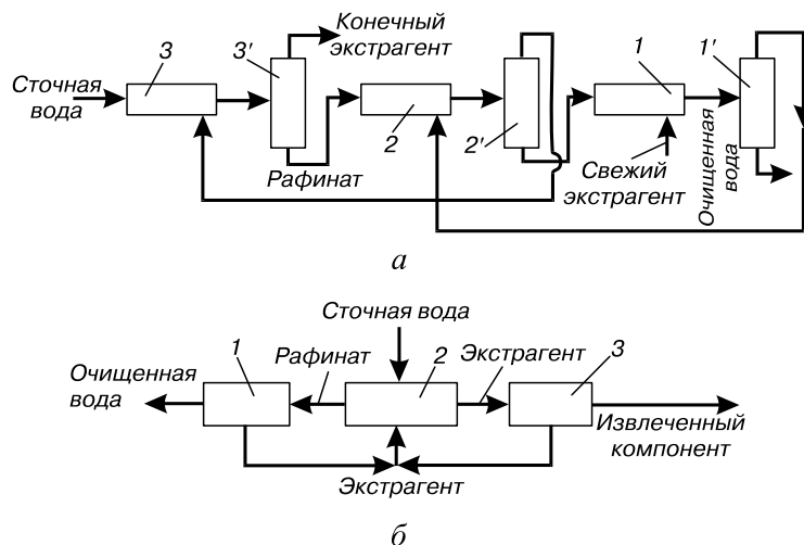
Рисунок 25.23.11 – Схемы процесса экстракции: а – многоступенчатого противоточного; 1–3 – смесители; 1'–3' – отстойники; б – непрерывного противоточного с регенерацией экстрагента из рафината и экстракта: 1 – система удаления экстрагента из рафината; 2 – колонна; 3 – система удаления экстрагента из экстракта
