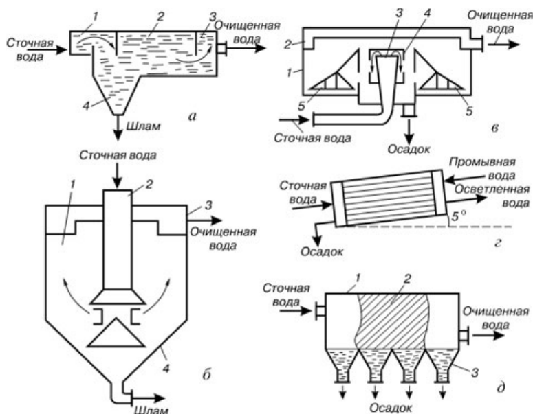
Рисунок 5.6 - Отстойники: а – горизонтальный: 1 – входной лоток; 2 – отстойная камера; 3 – выходной лоток; 4 – прямоток; б – вертикальный: 1 – цилиндрическая часть; 2 – центральная часть; 3 – желоб; 4 – коническая часть; в – радиальный: 1 – корпус; 2 – желоб; 3 – распределительное устройство; 4 – успокоительная камера; 5 – скребковый механизм; г – трубчатый отстойник; д – с наклонными пластинами: 1 – корпус; 2 – пластины; 3 – шламоприемник
