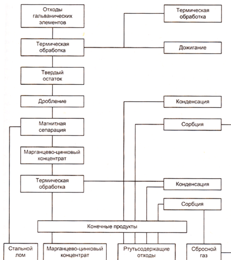
Рисунок 2.5 – Схема процесса демеркуризации отходов потребления и производства гальванических элементов
