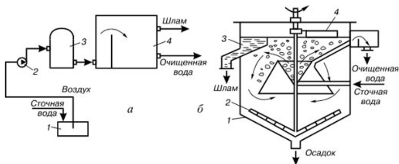
Рисунок 5.7 - Напорная флотация: а – схема напорной флотации: 1 – емкость; 2 – насос; 3 – напорный бак; 4 – флотатор; б – флотатор «Аэрофлотор»: 1 – камера; 2 – скребок; 3 – шламоприемник; 4 – поверхностные скребки
