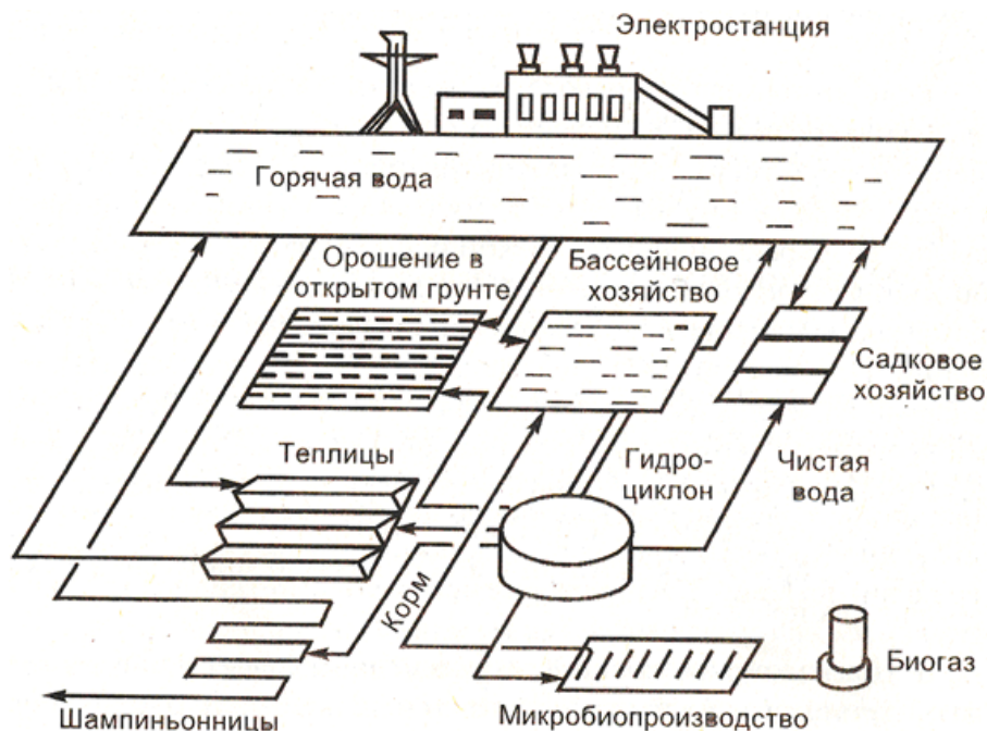
Рисунок 3.5 - Энерго-продовольственный комплекс на базе ТЭС
