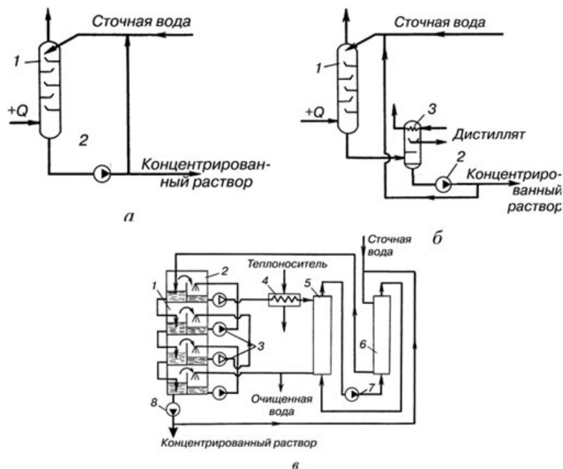
Рисунок 5.12 - Схемы выпарных установок: а-б – одноступенчатых контактных соответственно с испарением в камере контактного теплообменника и в адиабатной ступени: 1 – контактные теплообменники; 2 – насосы; 3 – адиабатный испаритель; в – с гидрофобным теплоносителем: 1 – ступень адиабатного испарителя; 2 – конденсатор смешения; 3, 7, 8 – насосы; 4 – подогреватель; 5–6 – контактные теплообменники
