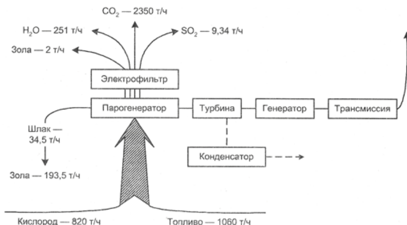
Рисунок 4.1 – Материальный баланс угольной ТЭЦ мощностью 2400 МВт
