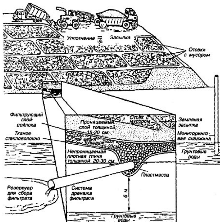
Рисунок 2.4 - Схема организации свалки с защитой грунтовых вод
